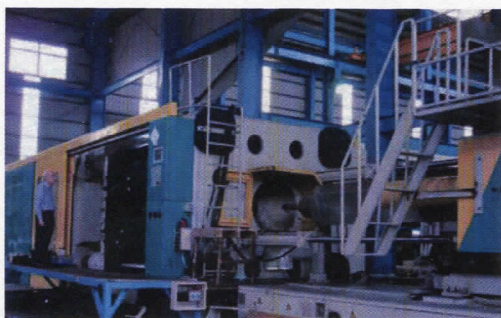
Pressa ad iniezione (4.000t) per la produzione di componenti di grosse dimensioni
